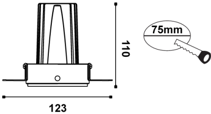
Plaster Trim
